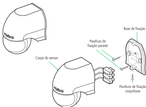
Fixação e instalação do sensor ESP 180
