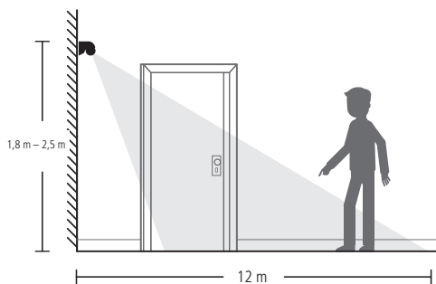
Altura e distância máxima de detecção
