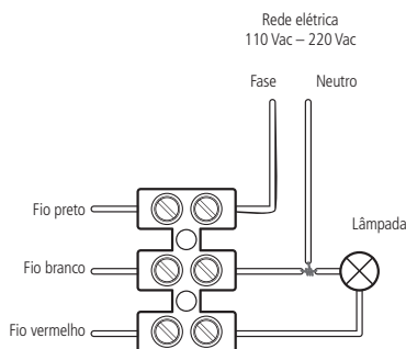
Conexões elétricas
